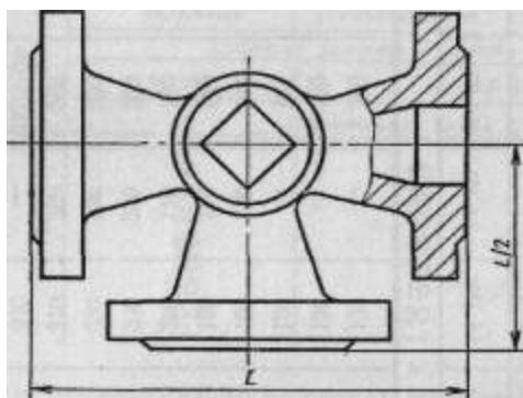
Кран трехходовой фланцевый
