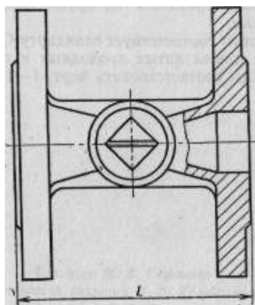
Кран проходной фланцевый
